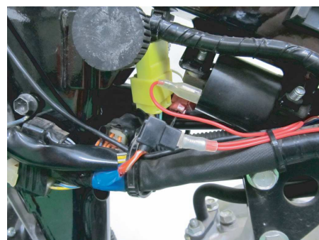
配線の接続先は、ECUカプラーハーネスと点火コイルハーネス
